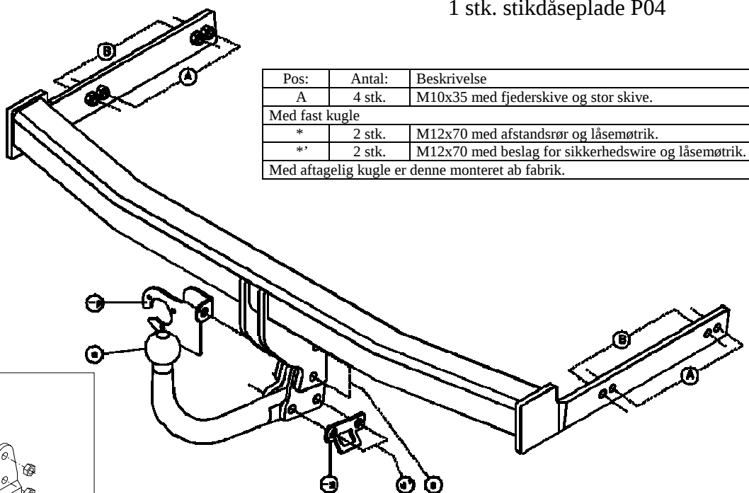
Montering af fast kuglestang.
