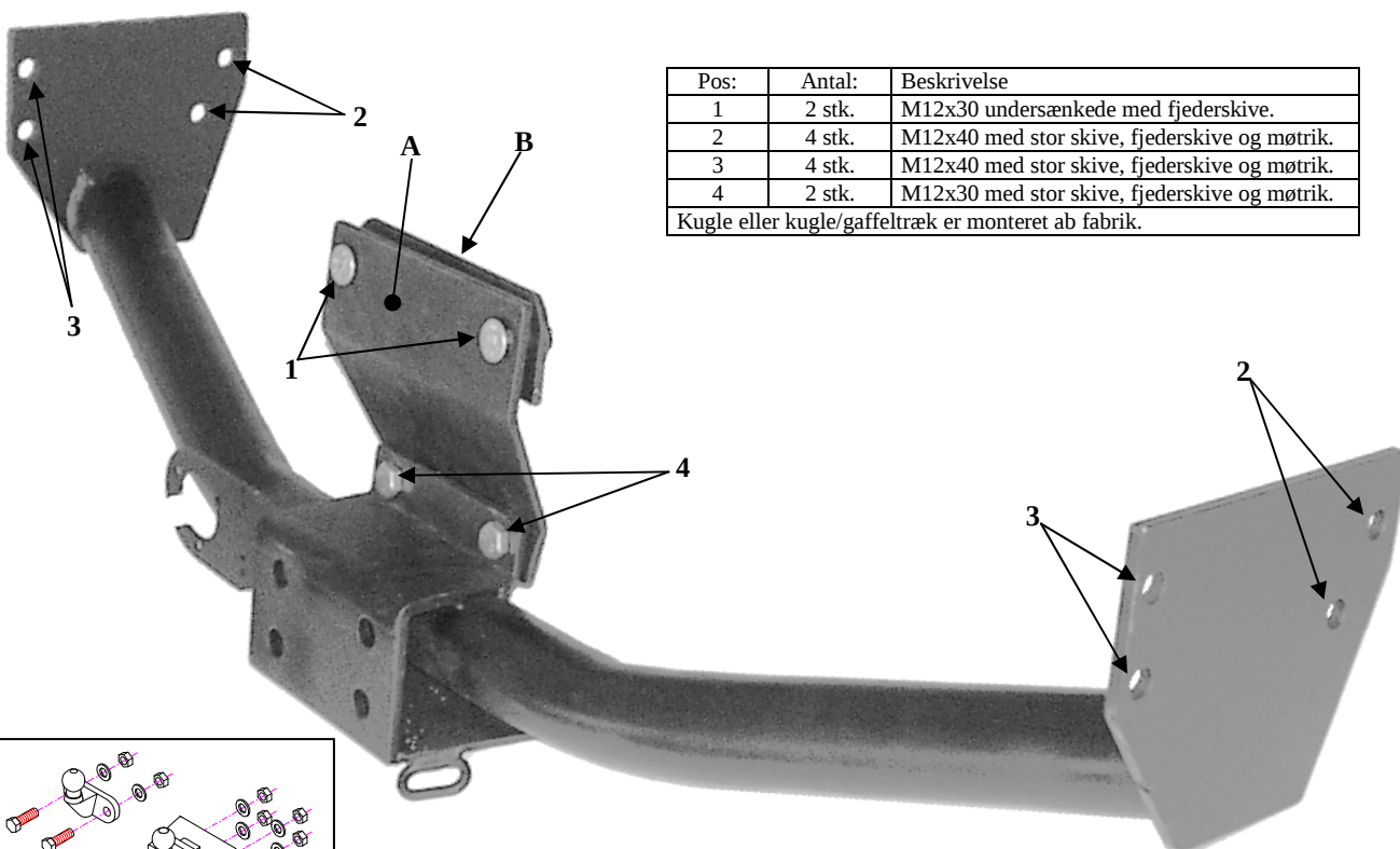
Montering af kugle - kugle/gaffeltræk.
