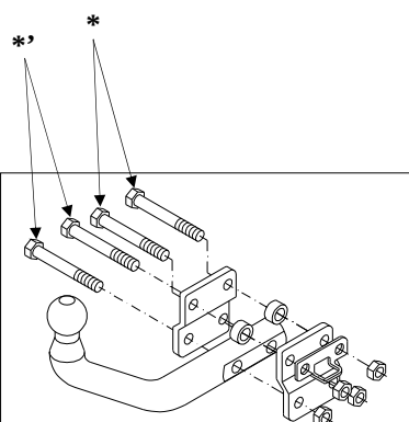
Montering af fast kuglestang.
