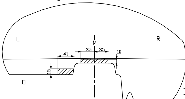
Tekening 1 - Citroën Sedan
