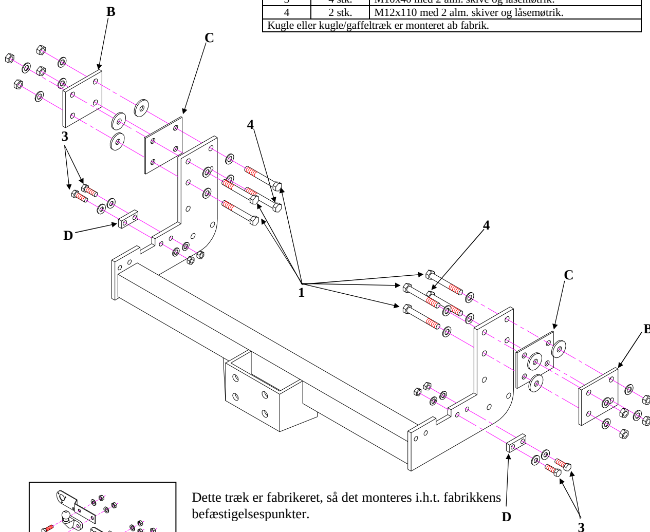
Montering af 8012 / 8079 på træk nr.: 2344
