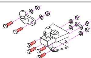
Montering af kugle - kugle/gaffeltræk.
