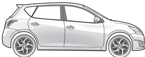
Pulsar
