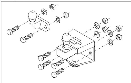
Kuglesystem til træk nr.: 1471 / 1471-8064
