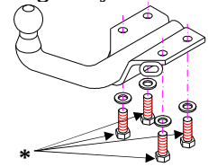
Montering af fast kugle - system T43
