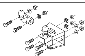
Montering af kugle - kugle/gaffeltræk.
